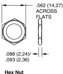
Hex Nut
